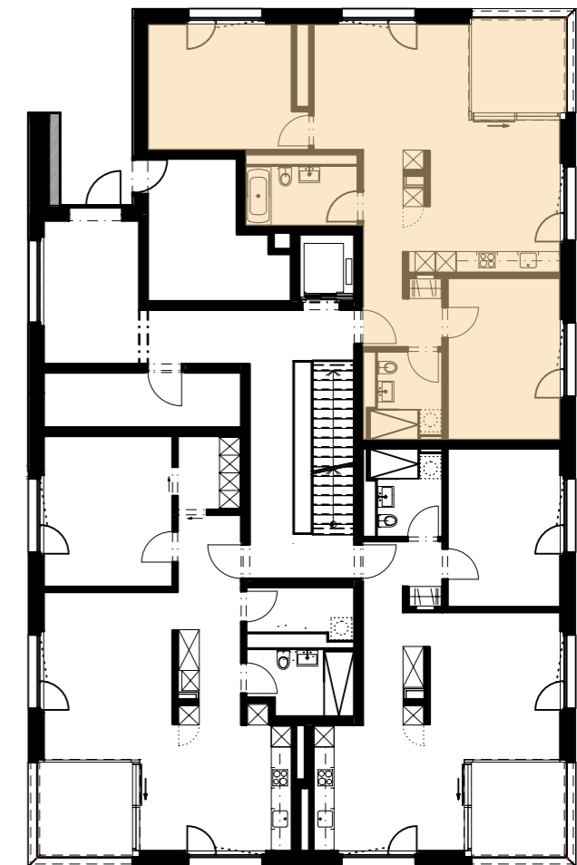
Wohnung Typ 1 1.OG (1x) 3.5 Zi
